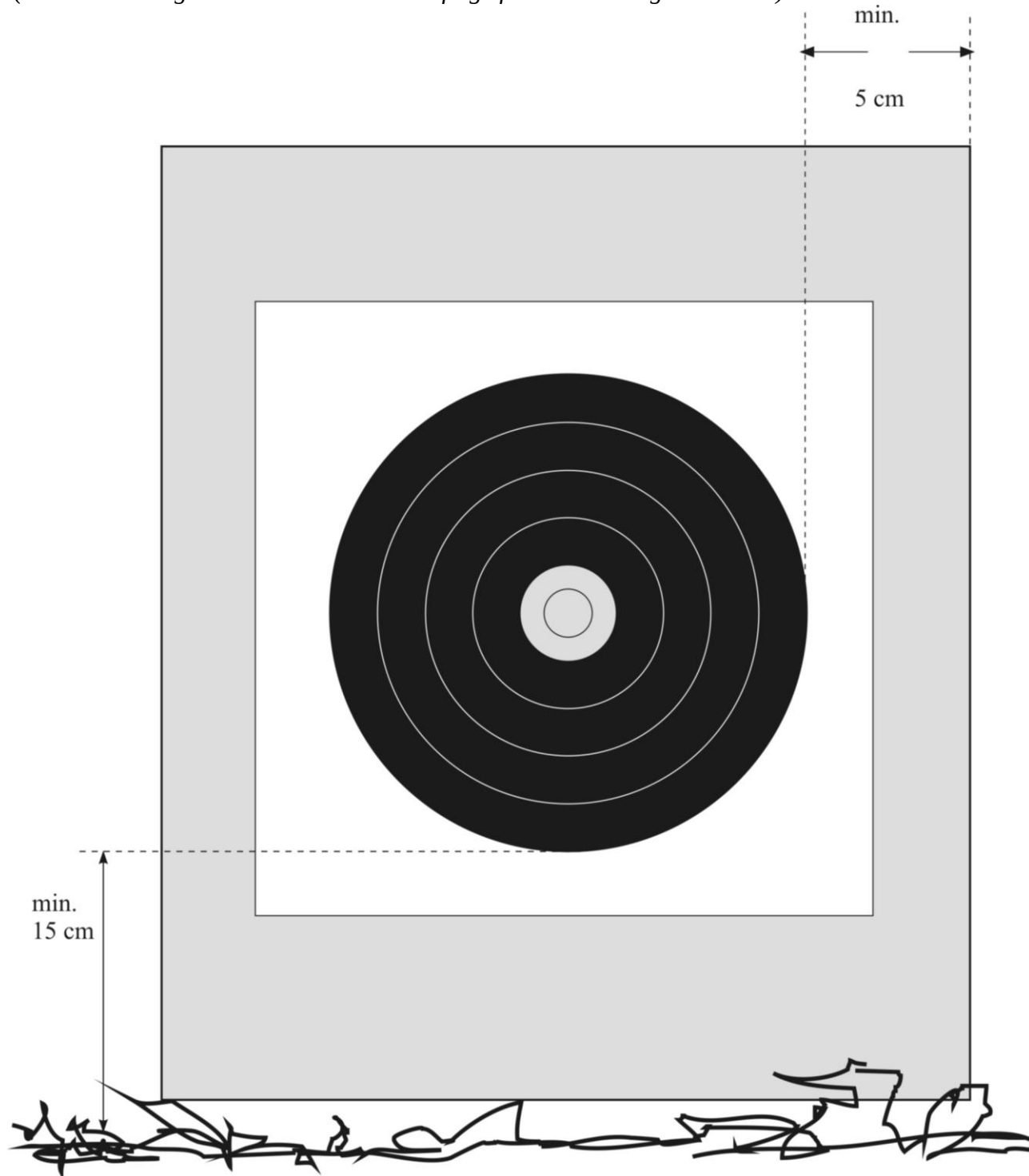
Abbildung 2: 80 cm- und 60 cm-Auflage für das Feldbogenschießen
