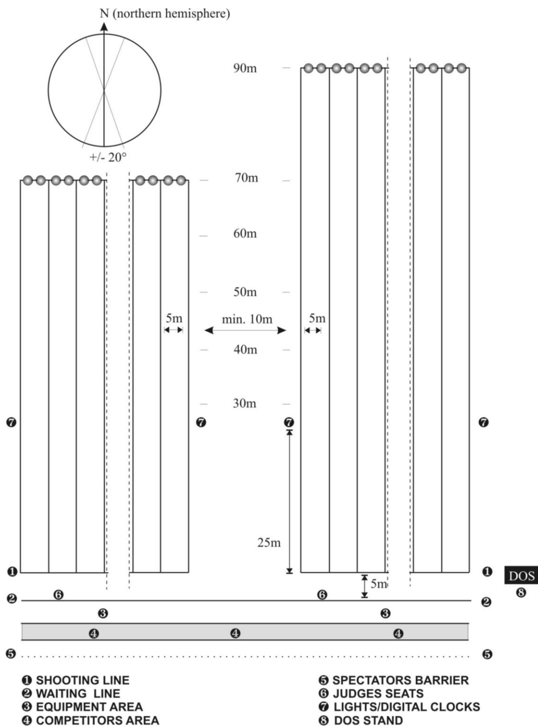
Abbildung 2: Anlage des Wettkampffelds
